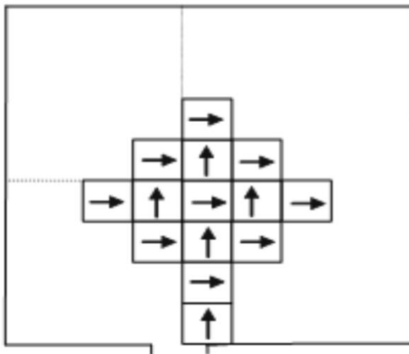
Parallel-/Schachbrett-Verlegung von Fliesen
