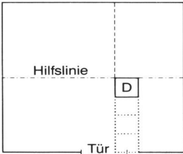
Anordnung der ersten Fliesenreihe
